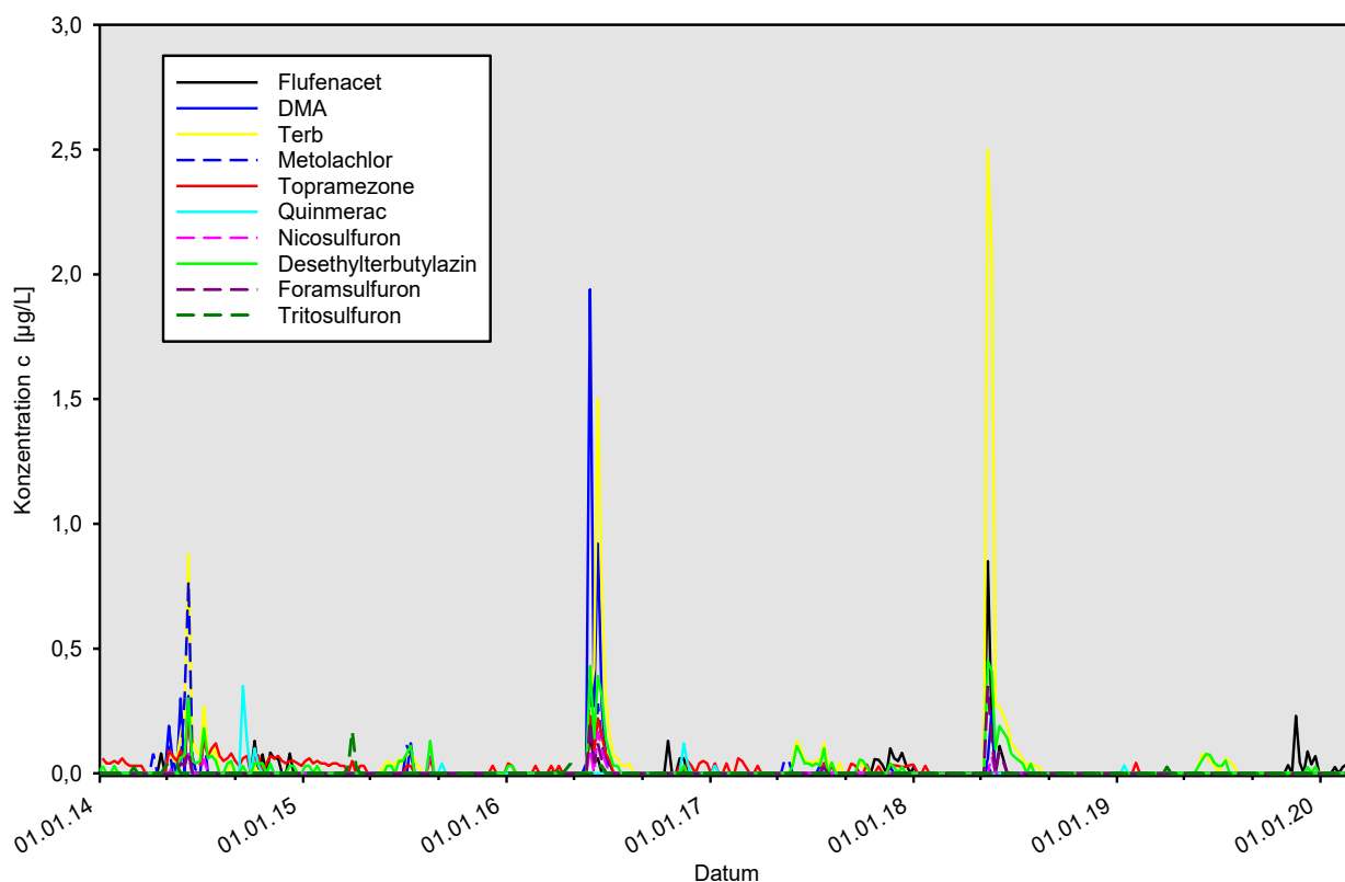
Bild 6: PSM-Befunde in der MP Funne (2014-2019)
