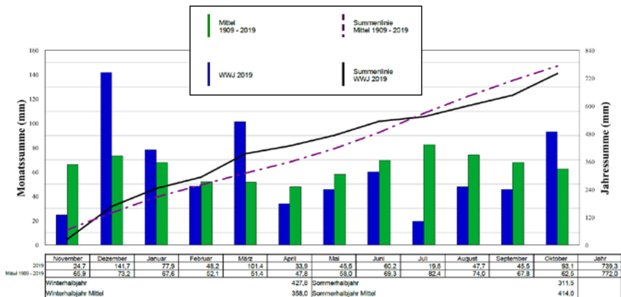
Bild 1: Niederschlagsmengen 2019 für das Wasserwerk Haltern (Grafik: GELSENWASSER AG)
