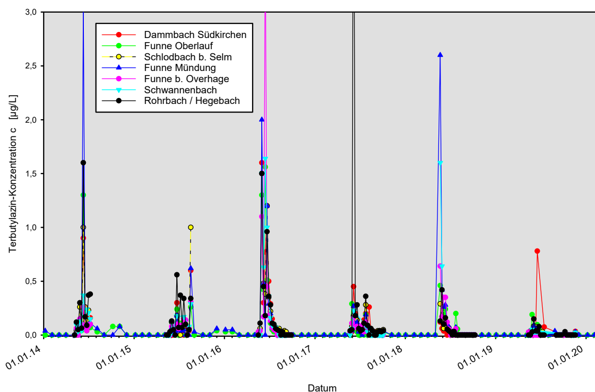
Bild 9: Terbutylazin-Befunde im Funne-Gebiet (2014-2019)
