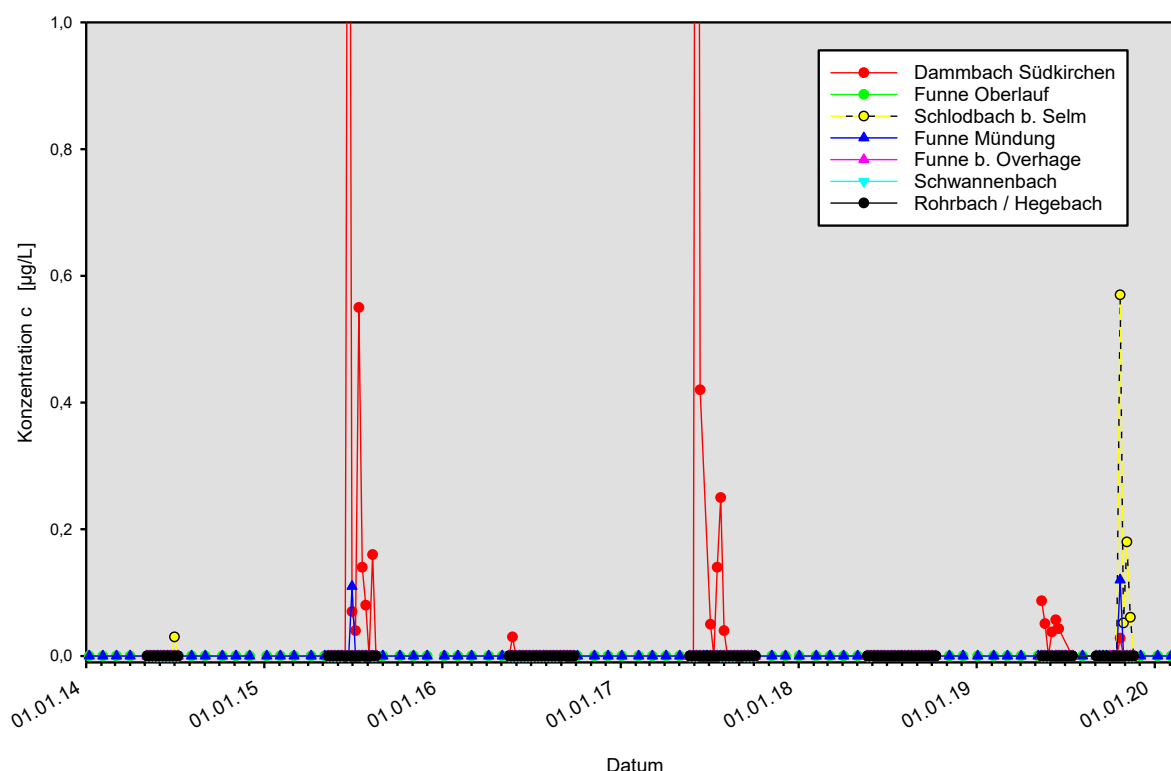
Bild 6: Metribuzin-Befunde im Funne-Gebiet (2014-2019)
